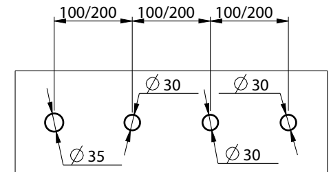
- Schema di foratura consigliato / Recommended drilling scheme
